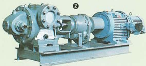
normal heating jackets for model RS pumps double enveloppe de réchauffage standard pour pompe série RS
