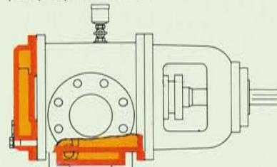
normal heating jackets for model RS pumps double enveloppe de réchauffage standard pour pompe série RS
