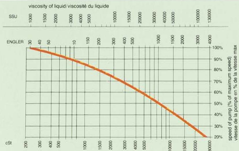
fig. 6 pump velocity as a function of the viscosity of the liquid / vitesse de la pompe en fonction de la viscosité du liquide pompé
